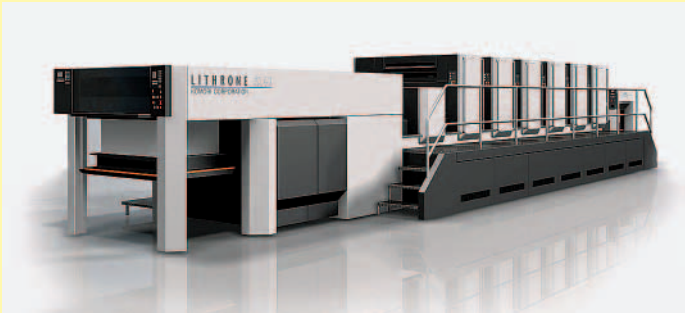
Die Lithrone SX 40 (Format 75 x 105 cm, 18 000 Bogen/h) von Komori, hier in der Sechsfarben-Version mit Lack (LSX-640+C).
